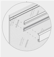
Ranura Continua
