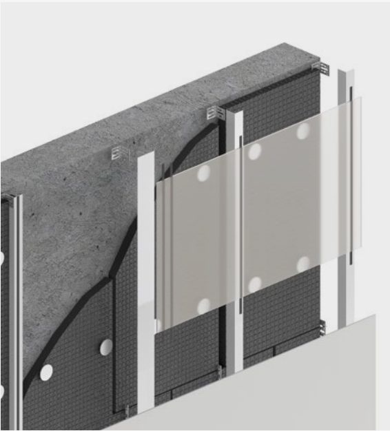
Sistema de anclaje químico
