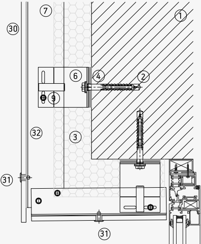
Dintel Dekton
