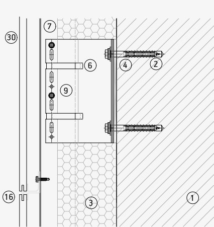
Junta horizontal
