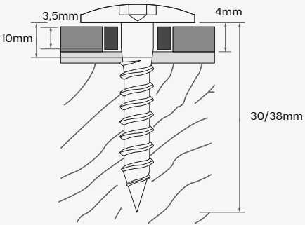
Punto fijo - Dekton 4 mm
