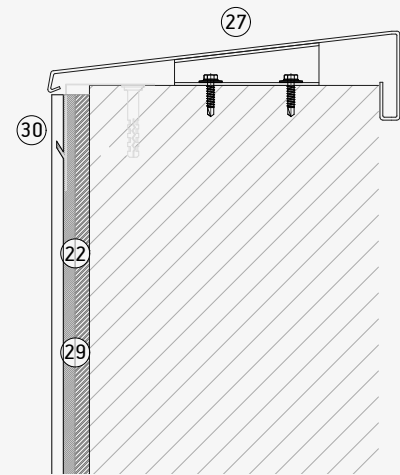
Junta horizontal
