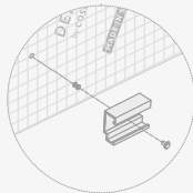
DKT1.Taladro destalonado TK (espesor=8/12 y 20 mm)
