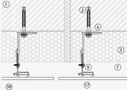
Junta de dilatación vertical
