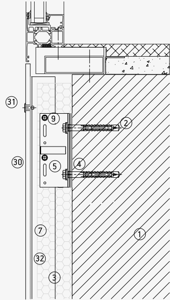
Arranque ventana
