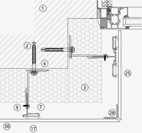
Jamba Dekton
