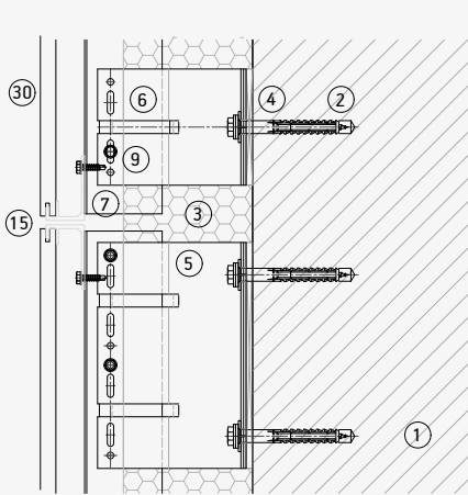
Junta entre perfiles
