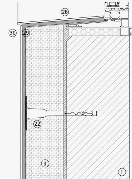
Vierteaguas con Dekton
