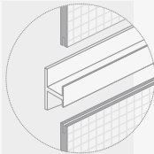
DKT2. Canto ranurado continuo Ancho 3/4 mm. (espesores= 12 y 20 mm)
