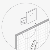
DKT3. Canto ranurado intermitente Ancho 3/4 mm. (espesores= 12 y 20 mm.)
