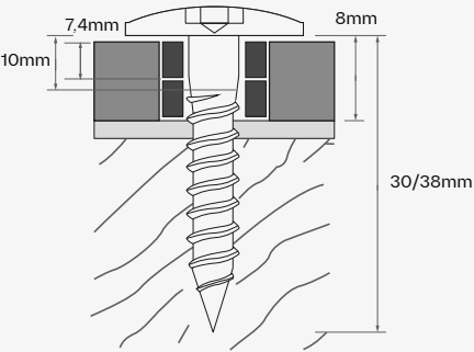
Punto fijo - Dekton 8 mm
