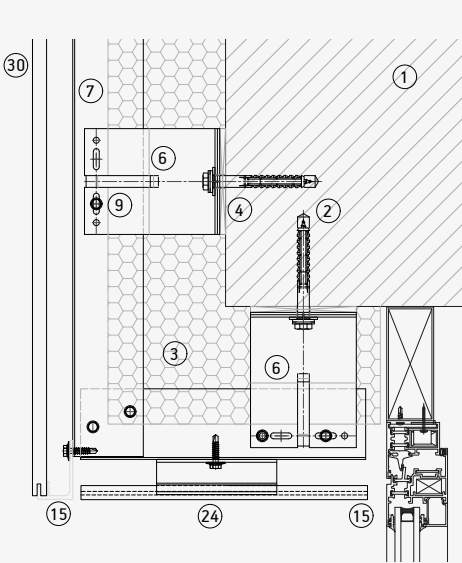
Dintel Dekton
