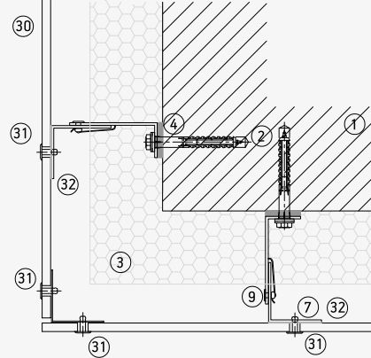
Esquina interior
