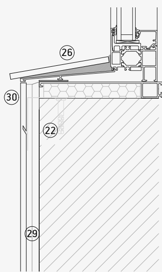
Vierteaguas con Dekton
