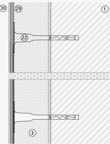
Junta de dilatación horizontal
