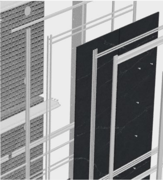
Detalle de capas del sistema
