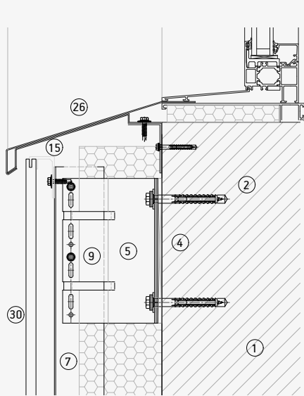
Alféizar de Ventana Metálico
