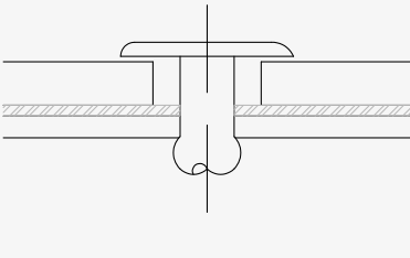
Punto móvil Dekton 4 mm
