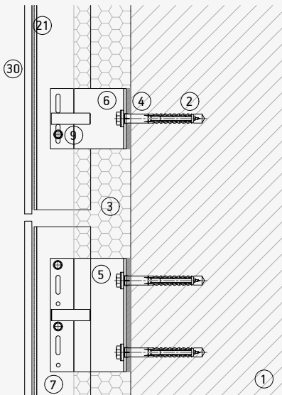
Junta horizontal
