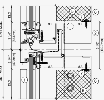
Junta Horizontal
