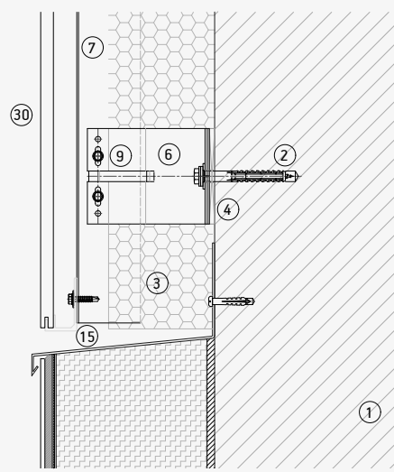
Arranque
