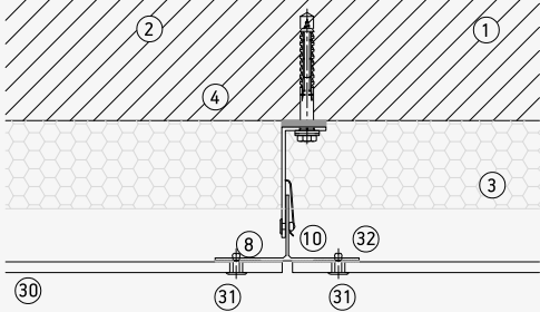
Junta vertical dilatación
