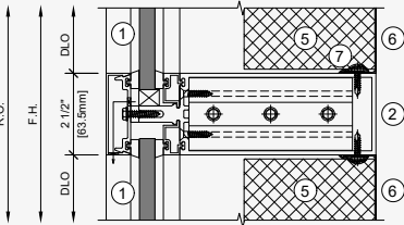
Junta Horizontal
