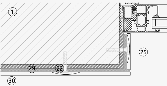
Jamba Dekton
