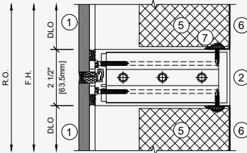
Junta Horizontal
