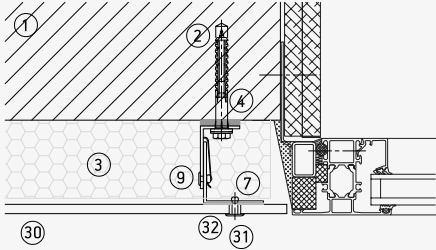
Lateral ventana
