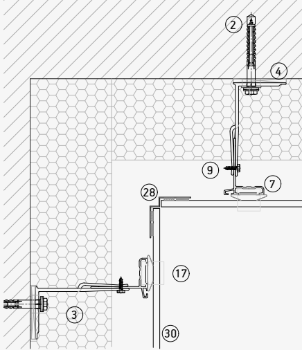
Esquina interior
