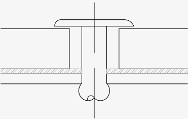
Punto móvil Dekton 8 mm
