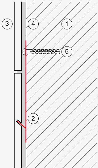
Detalle en sección de fijación oculta.
