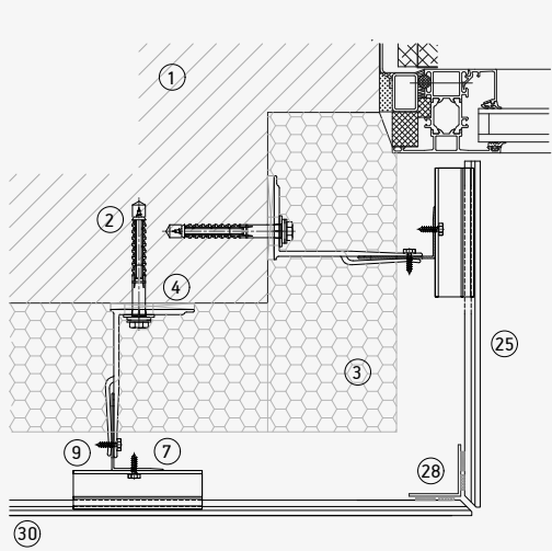
Jamba Dekton
