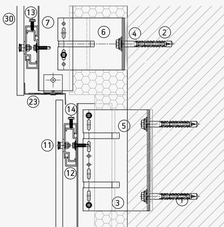
Opción junta entre perfiles
